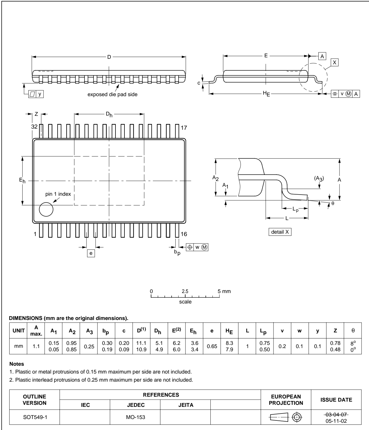
Fig 21. Package outline SOT 549-1 (HTSSOP32)
